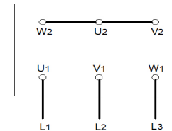
Y - bağlantı
