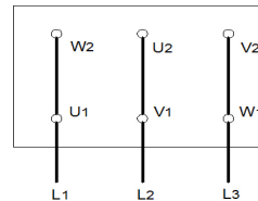
\Delta - bağlantı
